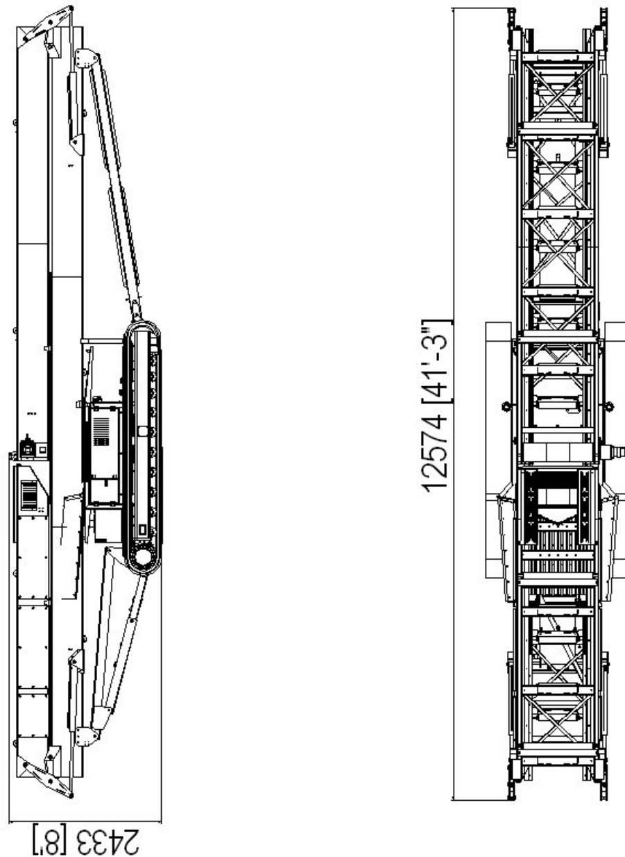
Fig. 2. TS80 Transportabmessungen
